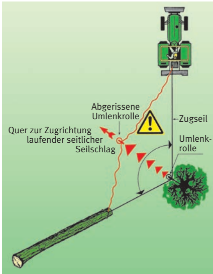
Gefahrenwinkel beim Einsatz der Umlenkrolle
